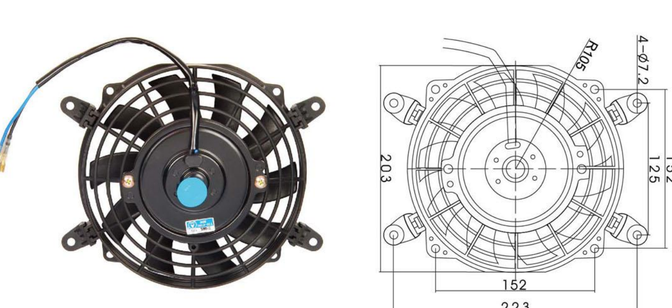
型号: (MODEL):SN81050-7S
