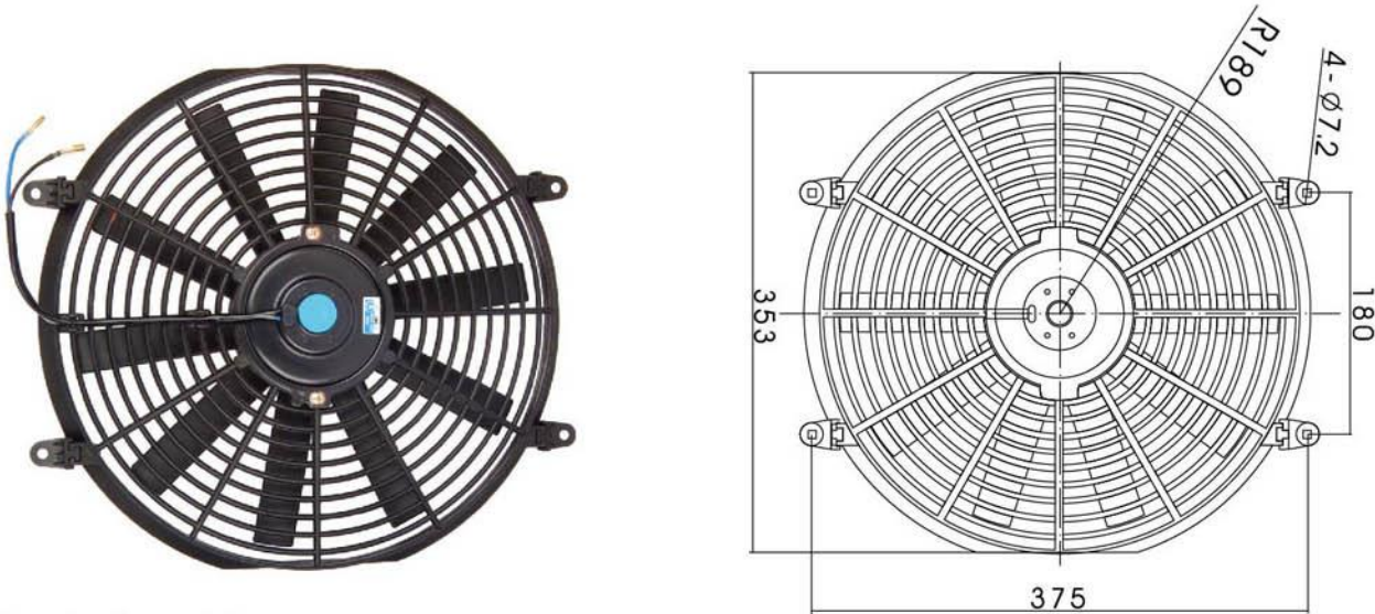
型号: (MODEL):SN81050-14L
