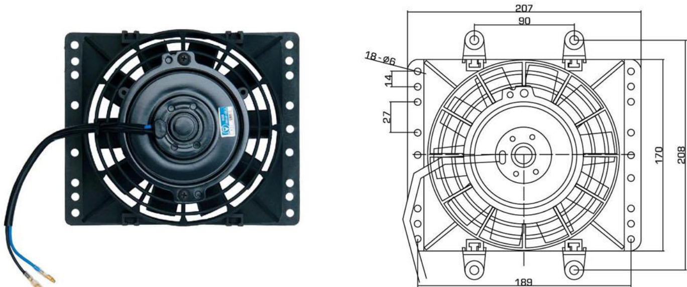
型号: (MODEL):SN81050-6B
