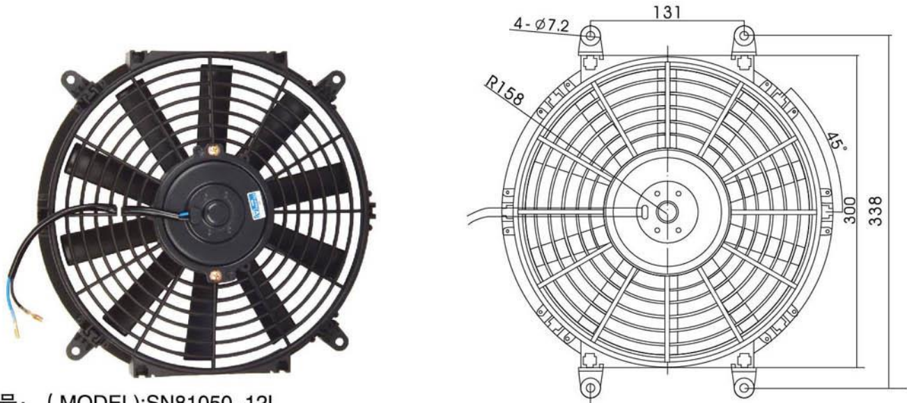
型号: (MODEL):SN81050-12L
