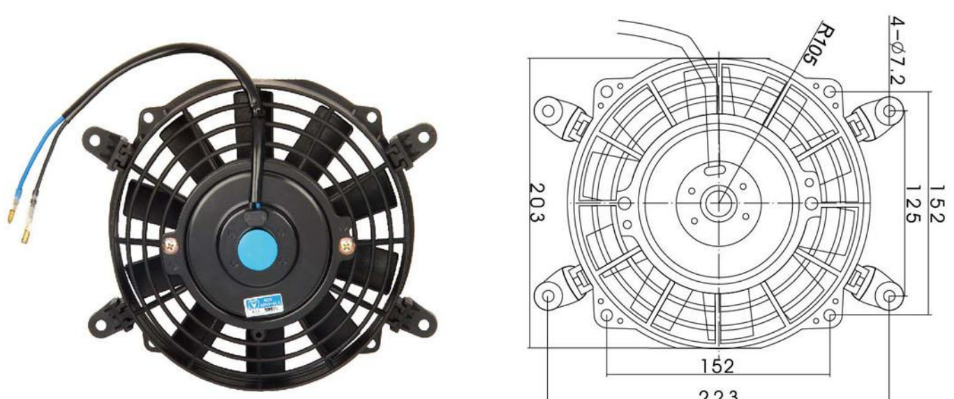
型号: (MODEL):SN81050-7L
