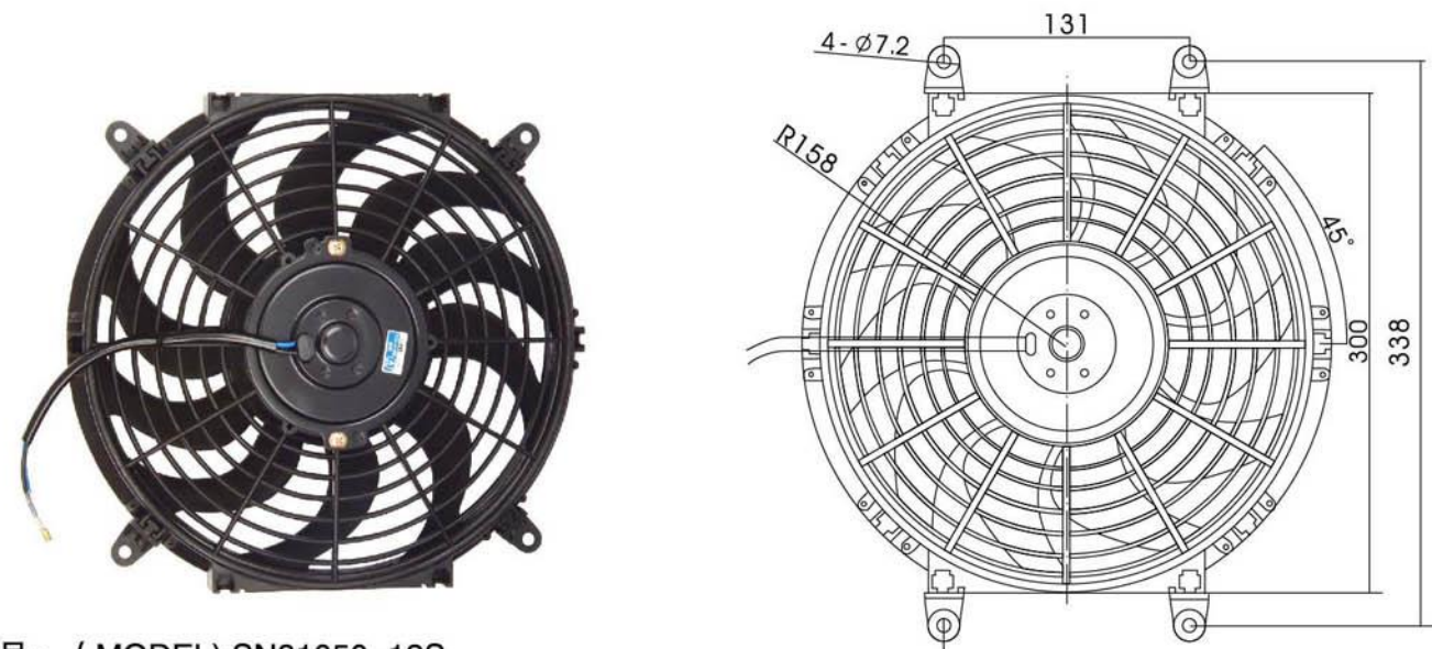
型号: (MODEL):SN81050-12S
